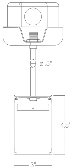
Pendant stem
